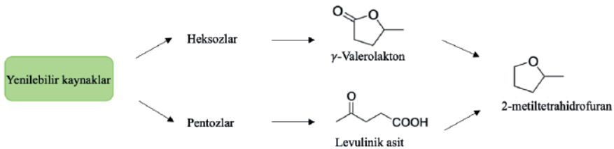
Şekil 16. 2-metiltetrahidrofuran sentezi
