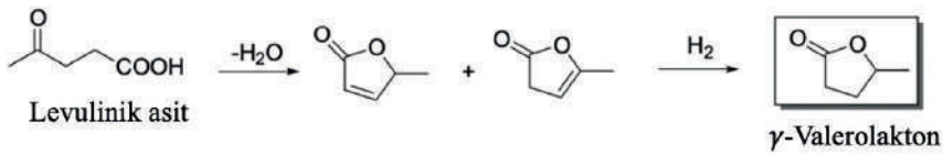
Şekil 15. Levulinik asitten GVL sentezi
